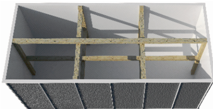
Versteifung des Skimmerbeckens und des Technischschachts
